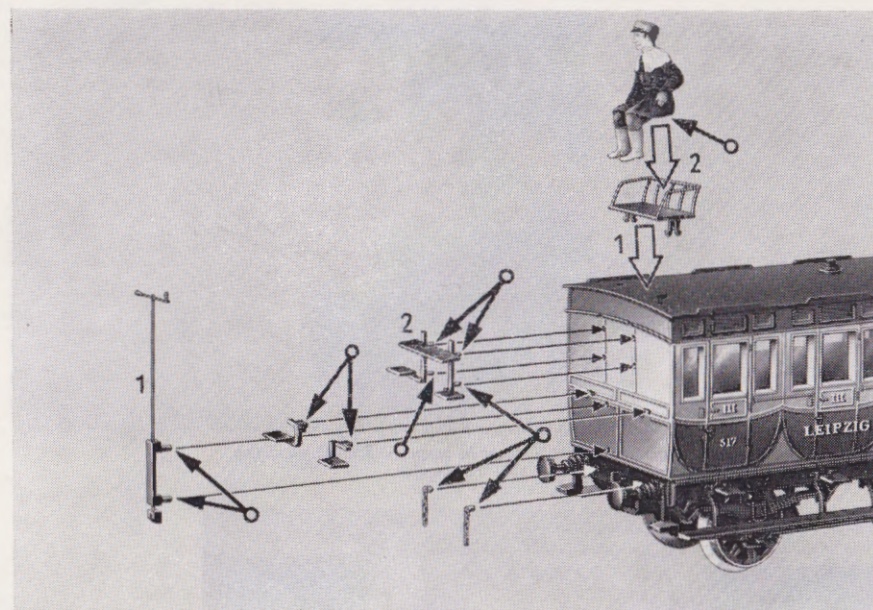
Zurüstteile einkleben • Glue in additional parts • Coller les pièces accessoires • Przykleić elementy wyposażenia dodatkowego • Детали оборудования вклеивать • Vlepte díly vybavení • Felszerelési darabokat beragasztani
