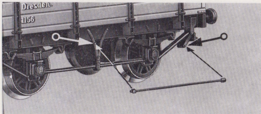
Zurüstteile einkleben • Glue in additional parts • Coller les pièces accessoires • Przykleić elementy wyposażenia dodatkowego • Детали оборудования вклеивать • Vlepte díly vybavení • Felszerelési darabokat beragasztani
